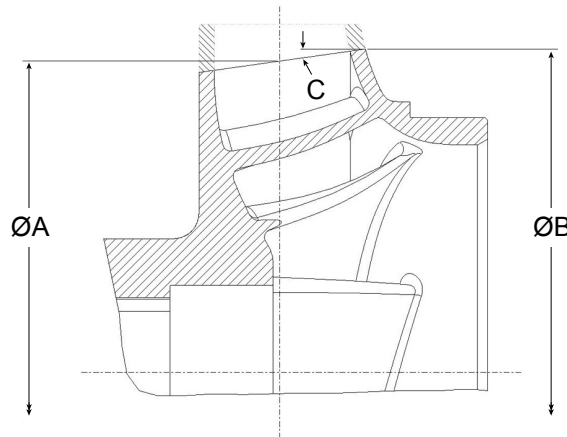
Figura 11: Recorte del impulsor 5x5x7B: incrementos de 0,125 pulg. (3,17 mm)
