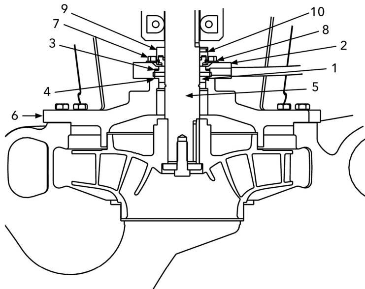
Figura 12: Sello externo
