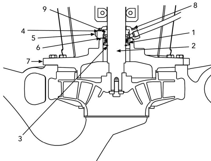
Figura 13: Sello interno
