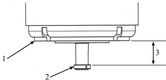
Figura 15: Fijación del anillo del cuello del motor para el motor 143-145TC e IEC
