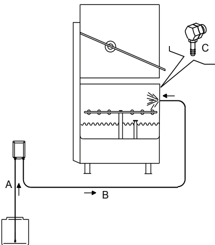
ANSCHLUSSPLAN Abb. 6
