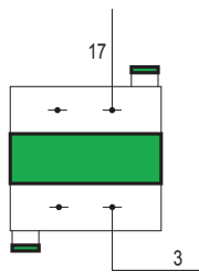
CONEXION PARA TIEMPOS 120 -180 SEG. PPG = 3-17 (SELECTOR TIEMPO)
