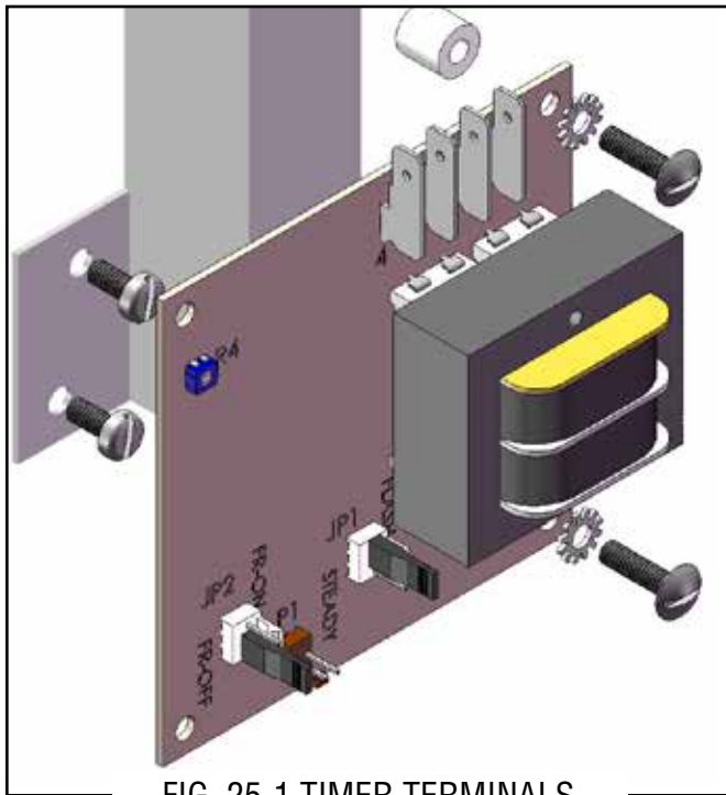
FIG. 25-1 TIMER TERMINALS
