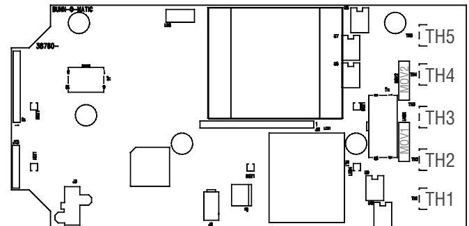
FIG. 12-2 TRIACS
