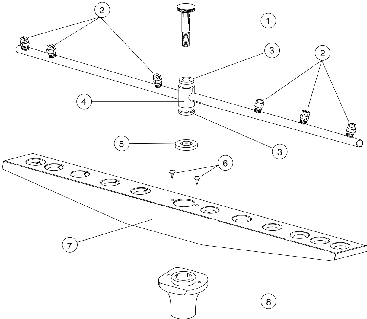
Figure 17 - Wash/Rinse Spray Arm Assembly Ensamblaje del brazo de rociar de Lavado/Enjuague
