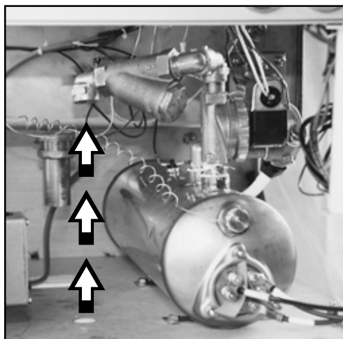
Figure 7 Hot Water Connection Conexión de agua caliente 3/4" NPT
