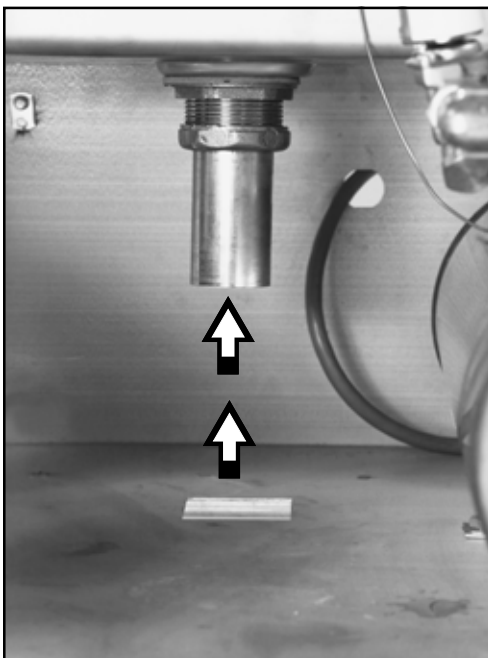
Figure 8 Drain Connection Conexión de desagüe 1-1/2" O.D.
