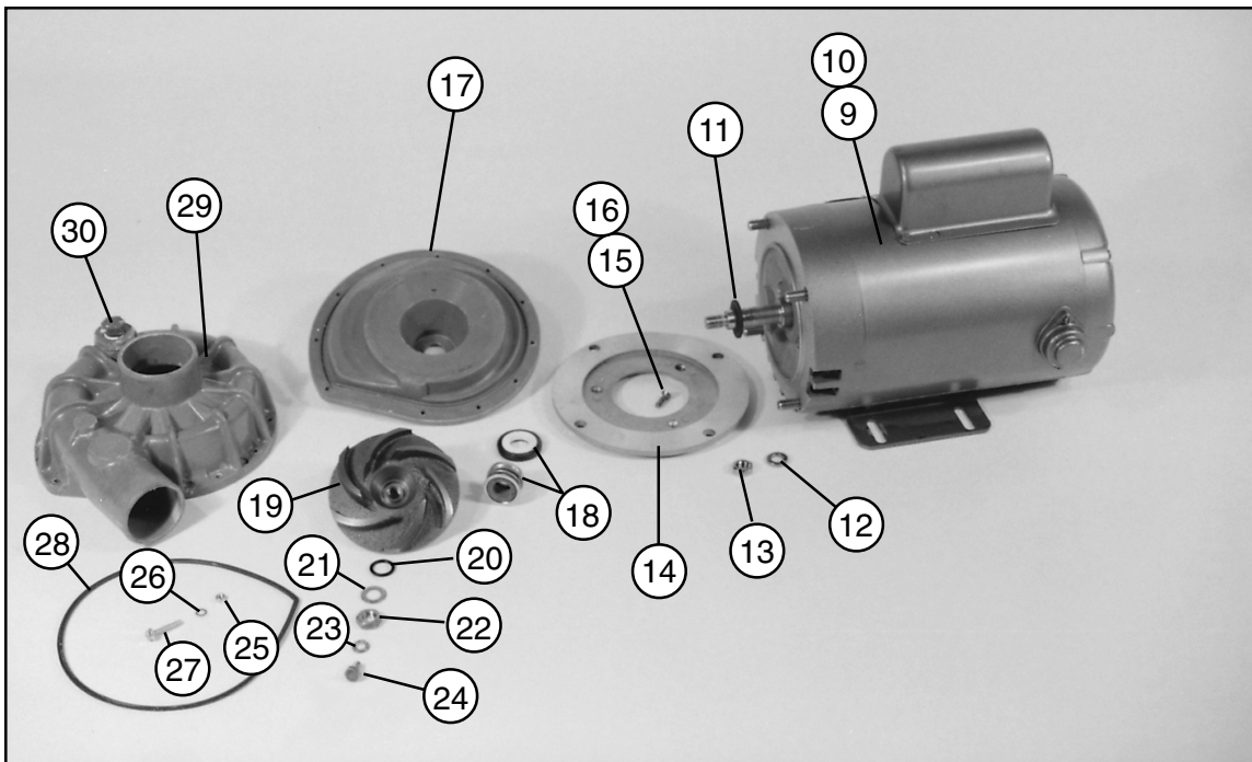
Figure 20 - Pump Assembly Ensamblaje de la bomba
