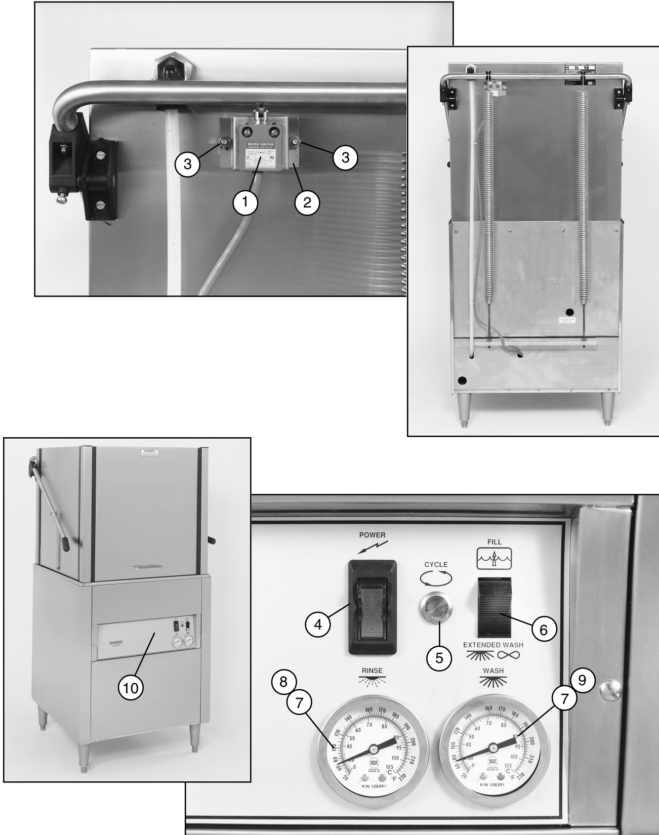
Figure 13 - Door Safety Switch and Instrument Panel Interruptor de seguridad de la puerta y panel de instrumentos
