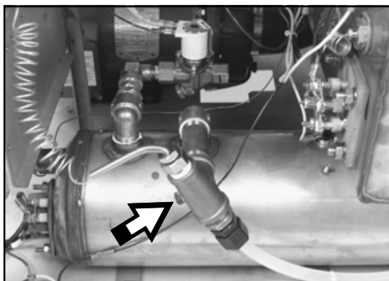
Figure 11 Rinse Aid Injection Point Punto de inyección auxiliar de enjuague 1/8" NPT
