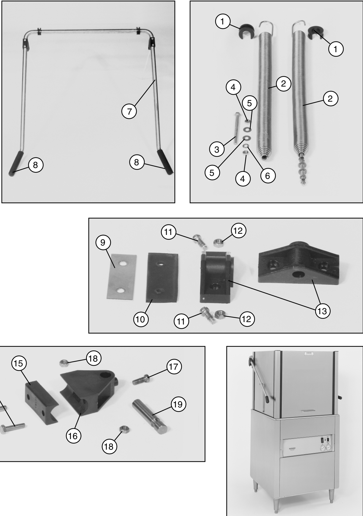
Figure 14 - Door Handle Assembly and Springs Ensamblaje y resortes de la manilla de la puerta
