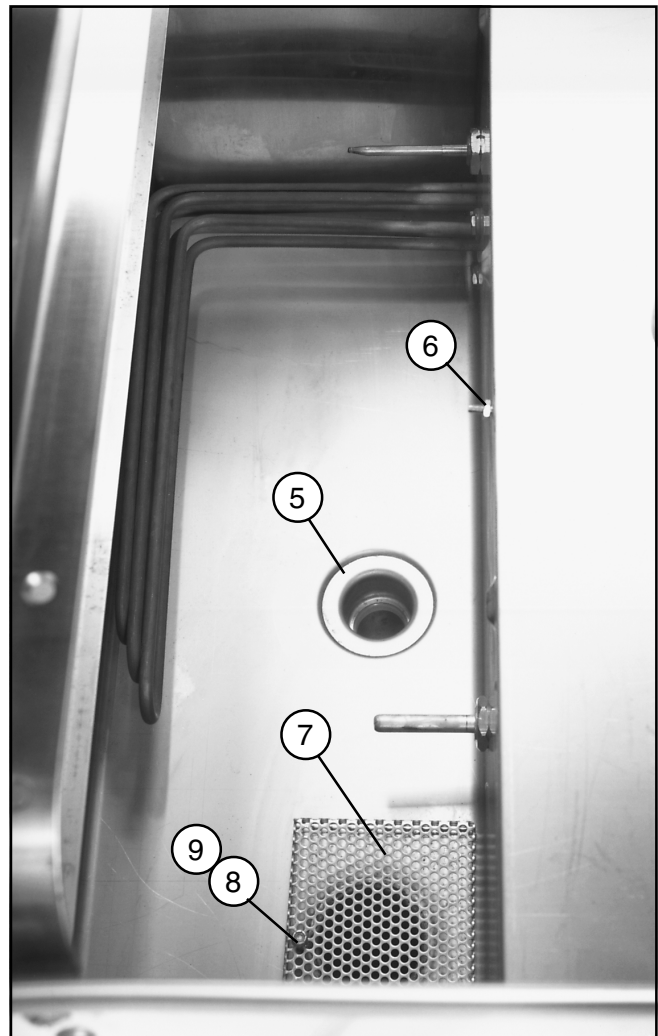
Figure 19 - Scrap Screens and Drain Assembly Ensamblaje de los filtros para desperdicios y del desague
