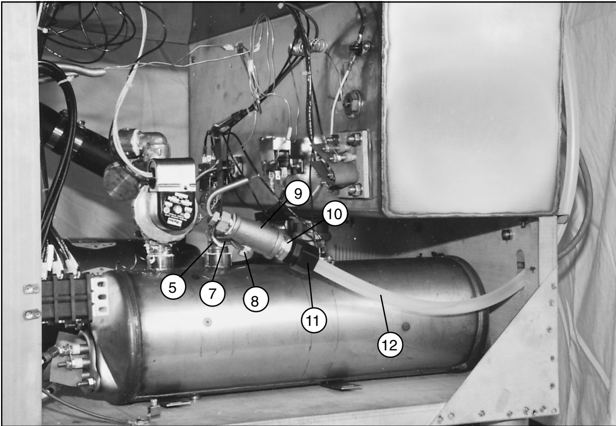
Figure 16 - Fill Piping Assembly Ensamblaje de las tuberías de llenado
