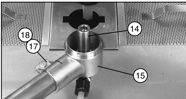
Figure 18 - Wash/Rinse Spray Piping Assembly Ensamblaje de las tuberías de rociado de Lavado/Enjuague
