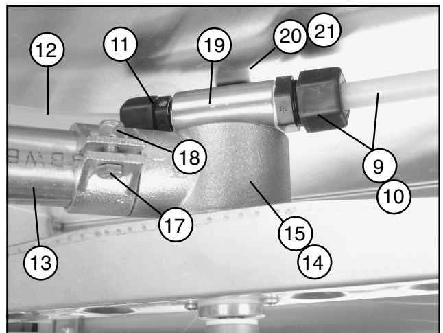
Figure 18 - Wash/Rinse Spray Piping Assembly Ensamblaje de las tuberías de rociado de Lavado/Enjuague
