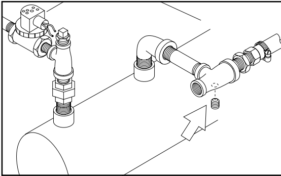
Figure 11 Rinse Aid Injection Point Punto de inyección auxiliar de enjuague 1/8" NPT
