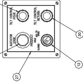
OPTIONAL ITEM
