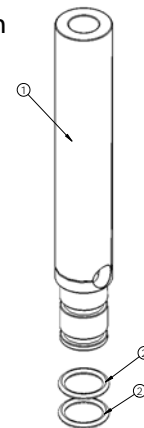
Low overrun carb tube (W0472060)
