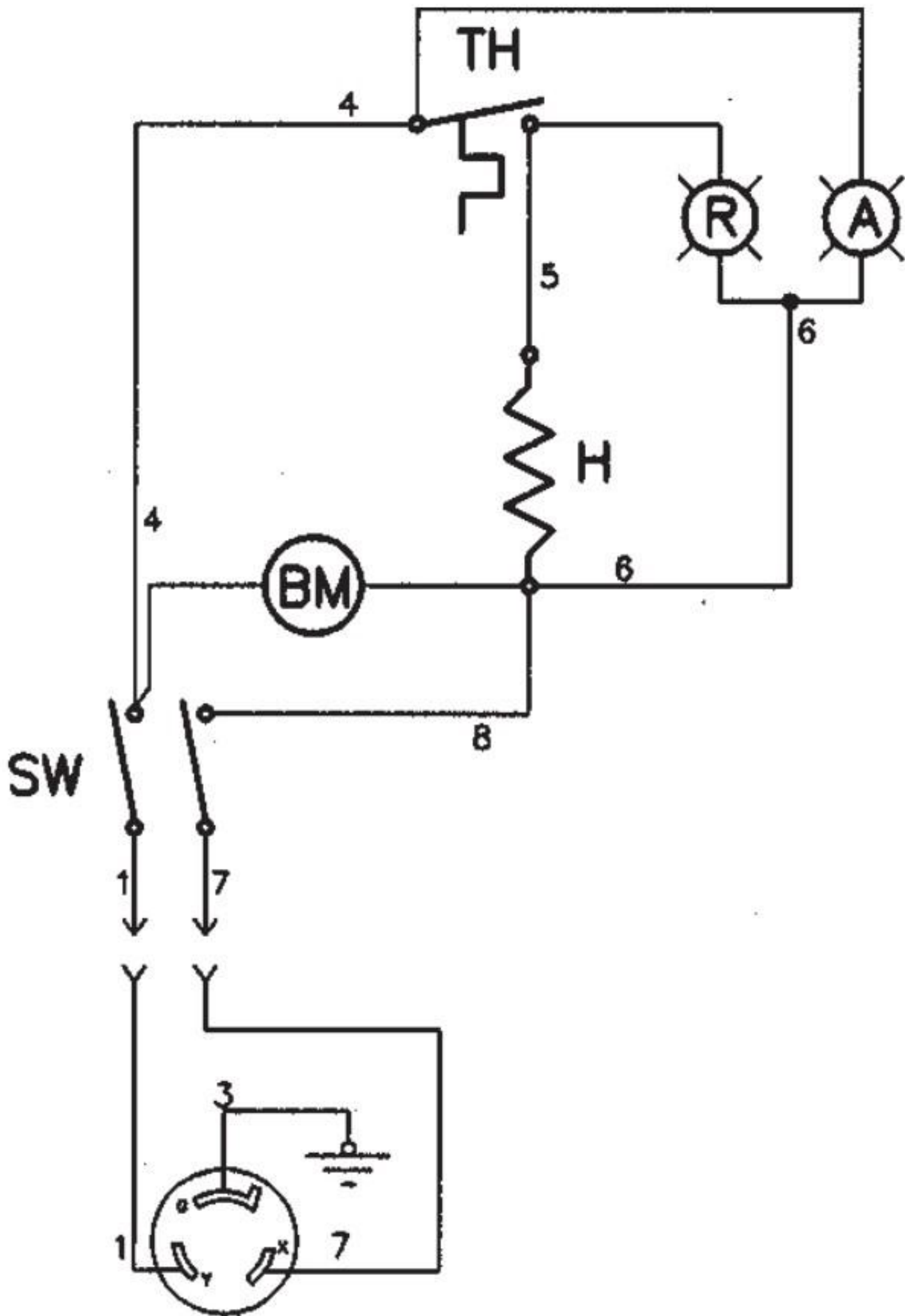
L6-15R (240V)
