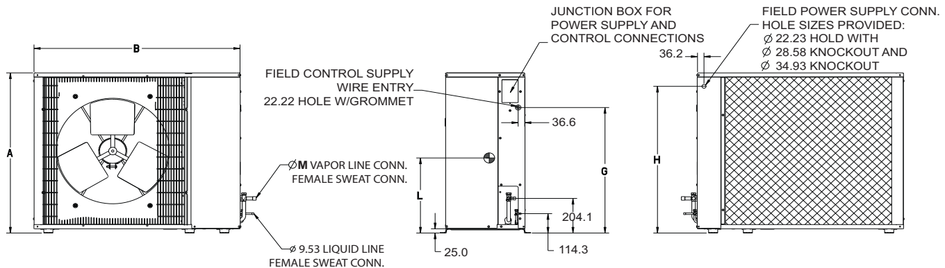
Fig. 5 — Dimensions
