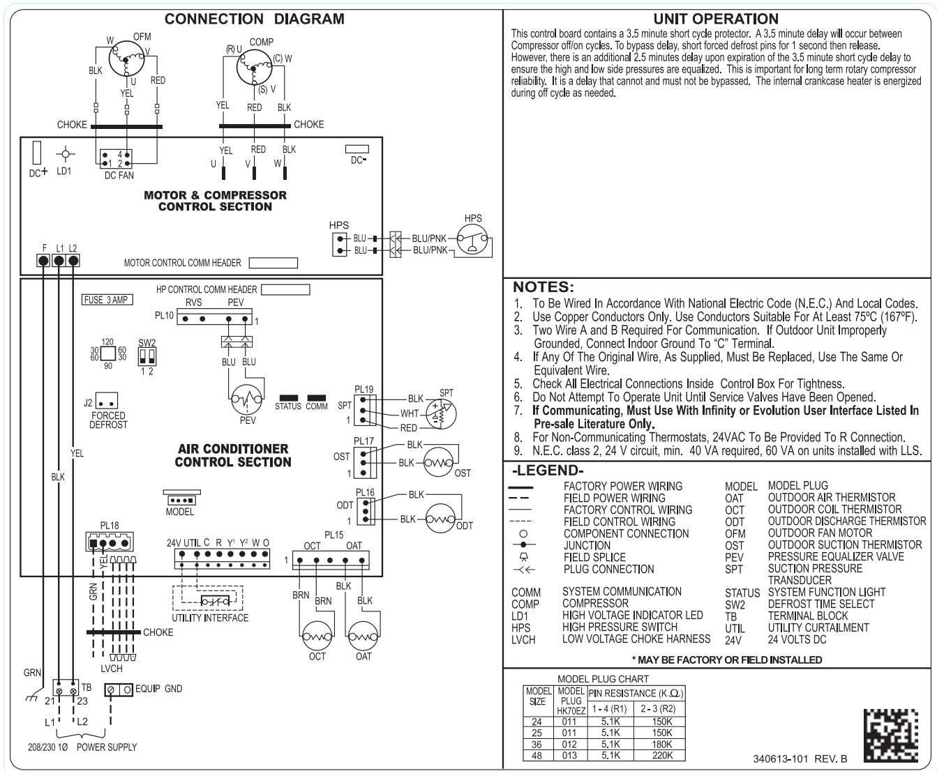
Fig. 1 – 24VNA9 208/230-1
