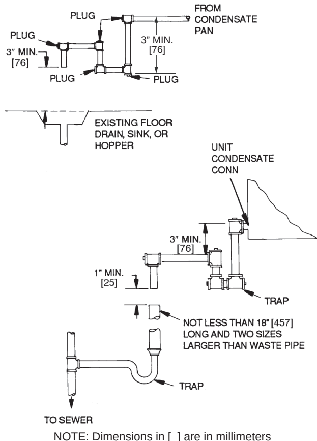
Fig. 12 - Condensate Drains
