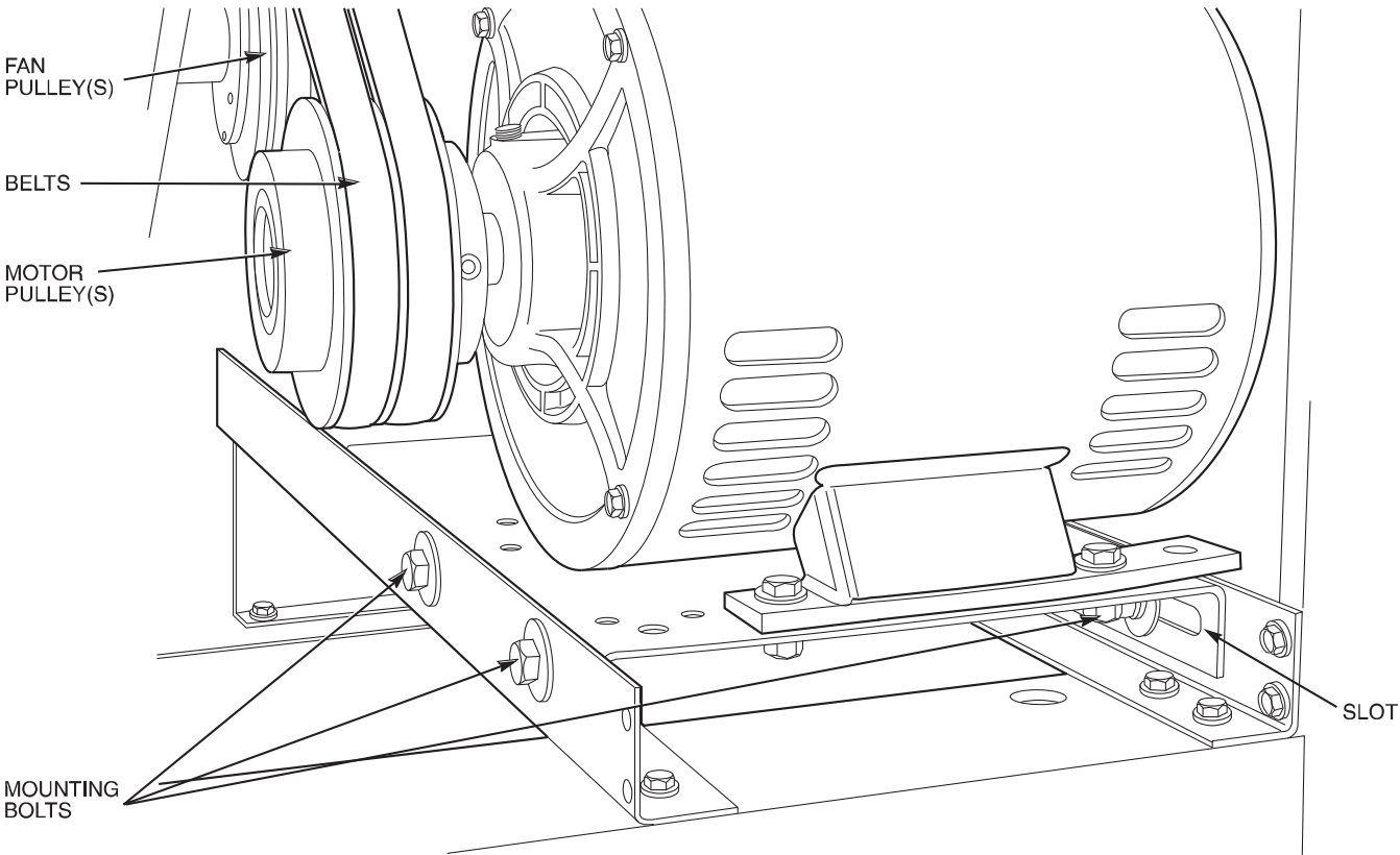
Fig. 24 - Fan Motor Mounting
