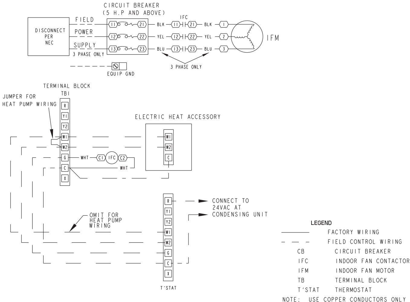
Fig. 17 - Unit Wiring
