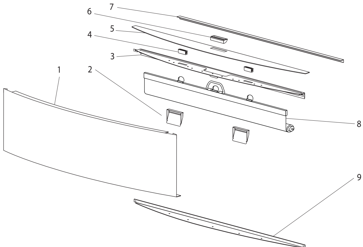
Figure: PL-1 Front Décor Panel
