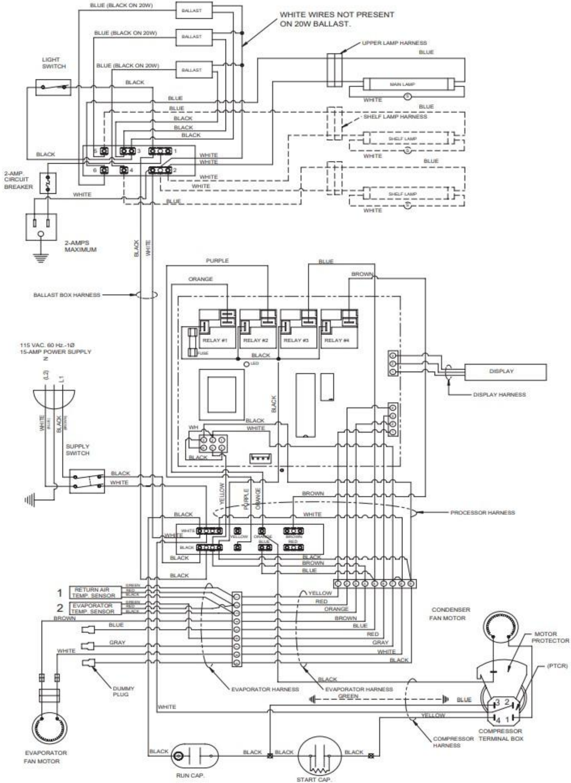
WIRING DIAGRAM-DISPLAY, MED-TEMP. 00-0217-00
