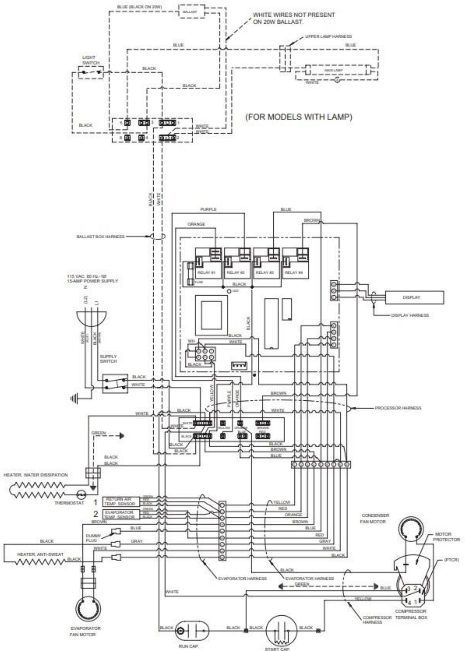
WIRING DIAGRAM-OPEN, MED-TEMP. 00-0219-00
