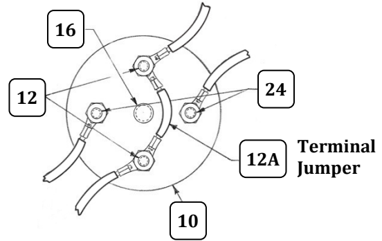
Terminal Wiring
