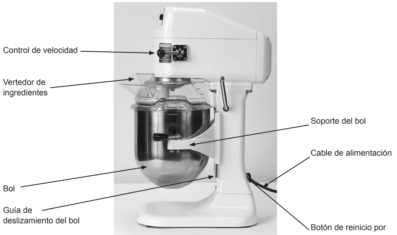
VISTA LATERAL
