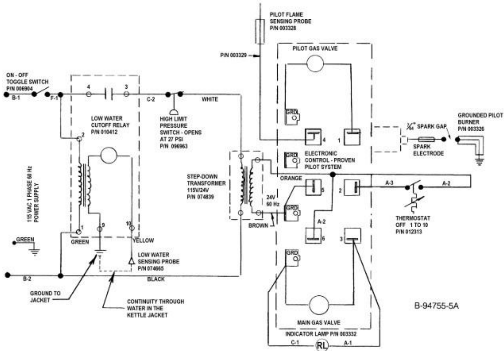
HH/4E Spark Ignition, Type QHL-1
