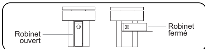
Positions du robinet de vidange
