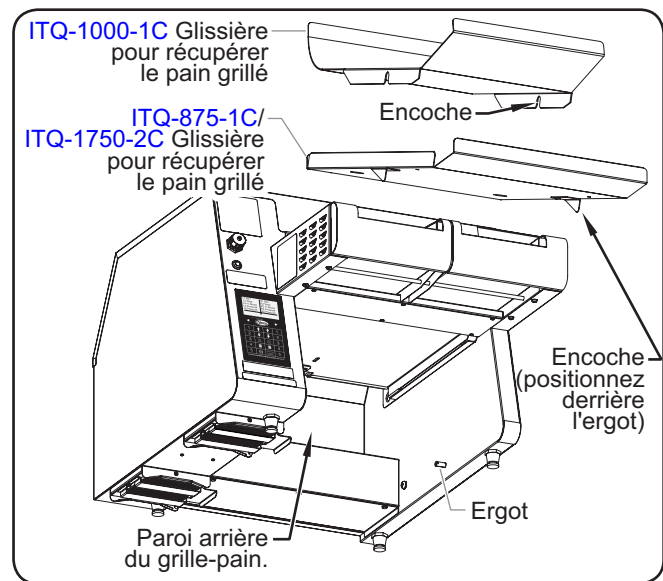
Installation de la glissière pour récupérer le pain grillé
