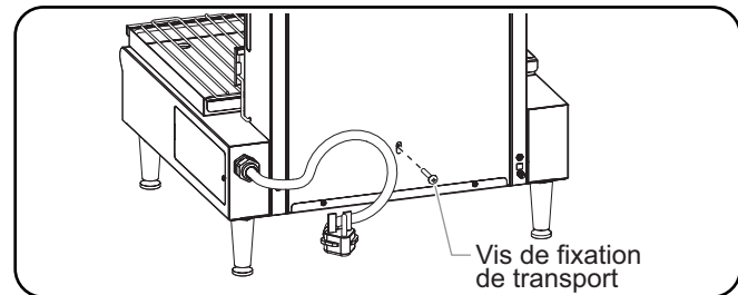
Vis de fixation de transport
