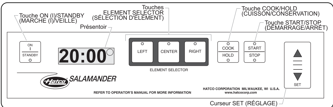
Panneau de commande de l'appareil Salamander
