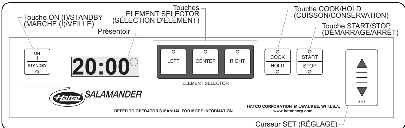
Panneau de commande de l'appareil Salamander
