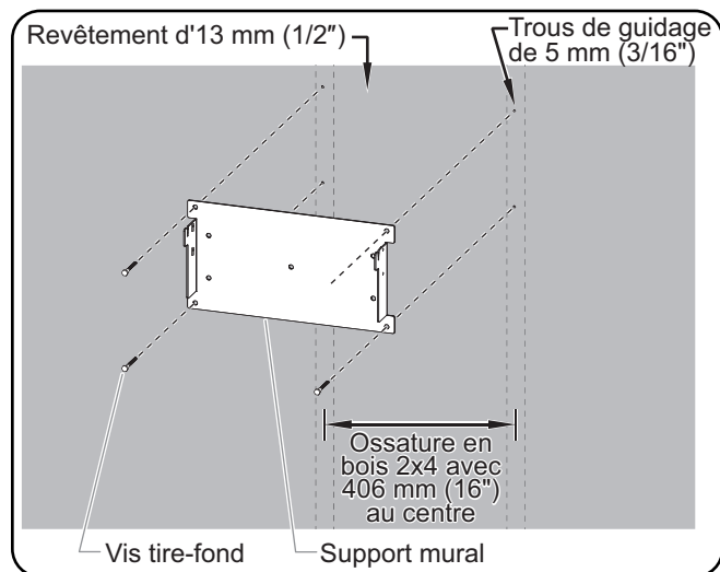
Fixation du support mural
