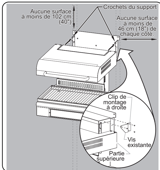
Accrochage de l'appareil
