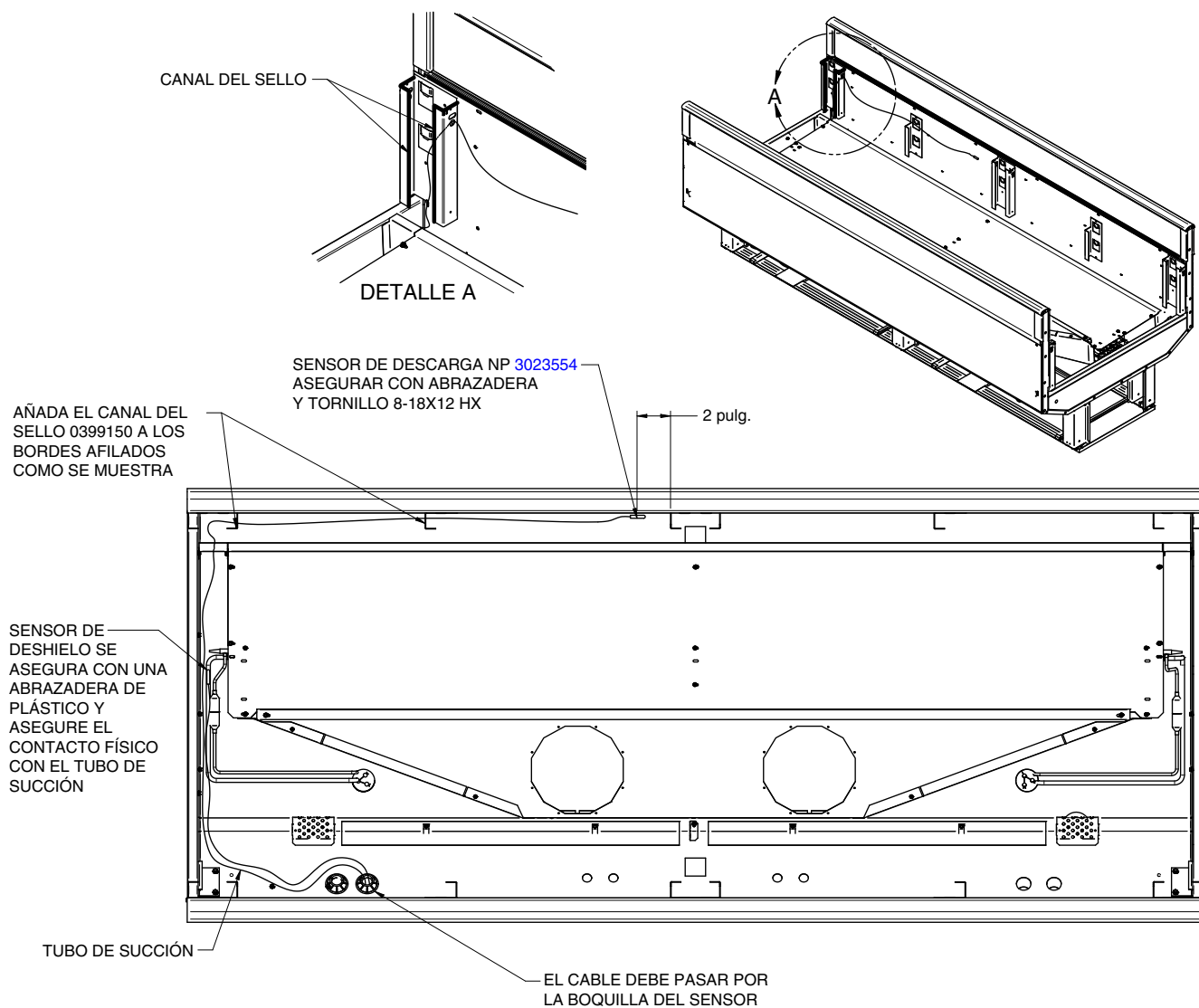
Ubicación del sensor - FNGSC8A
