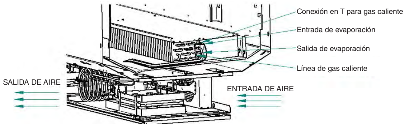
Circuito de refrigeración N° 2 (lado derecho)
