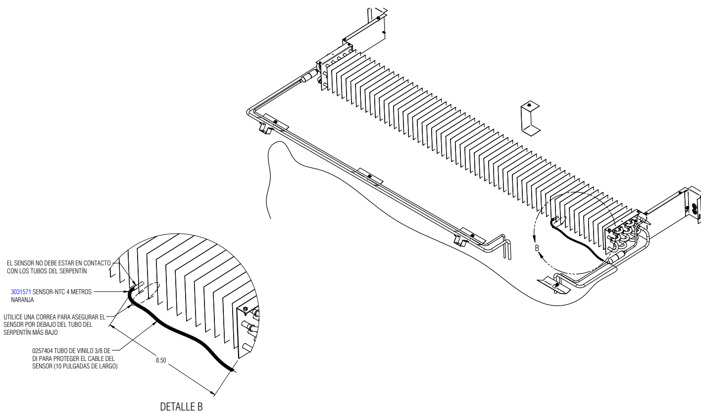
Ubicación del sensor del deshielo - FNGSC6A
