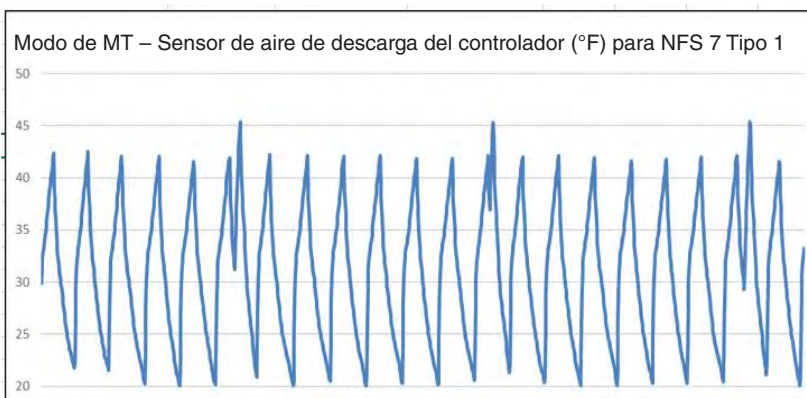
Ejemplo de FNGSC8A (temperatura media)
