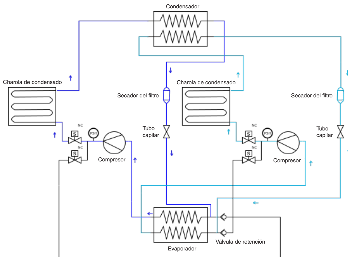
Diagrama del sistema - Modo de refrigeración (FNGSC6A)
