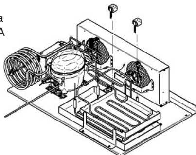
Unidad condensadora FNGSC8A, FNGSC4A
