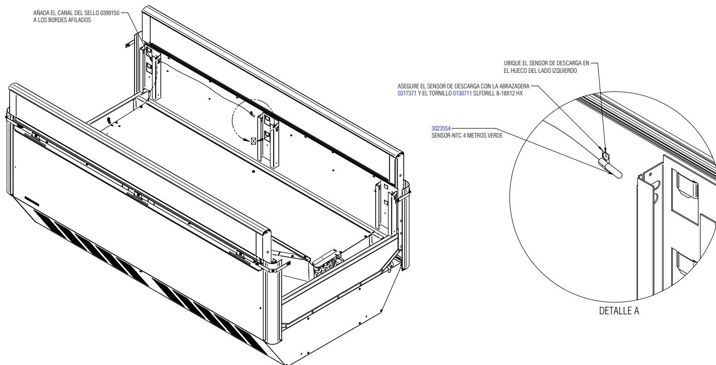
Ubicación del sensor del aire de descarga - FNGSC6A
