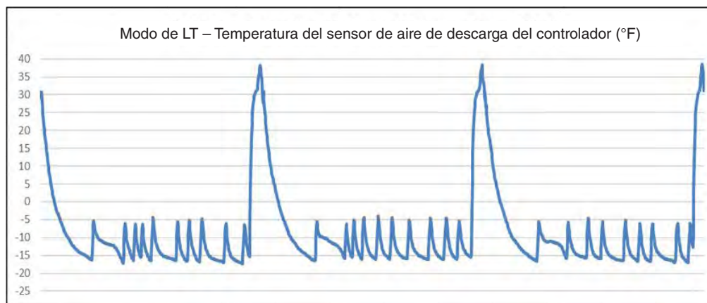
Ejemplo de FNGSC8A (temperatura baja)
