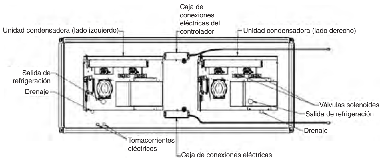
Distribución del compartimiento de la maquina
