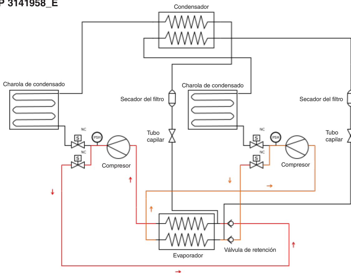
Diagrama del sistema — Modo de deshielo —Derivación de gas caliente (FNGSC6A)
