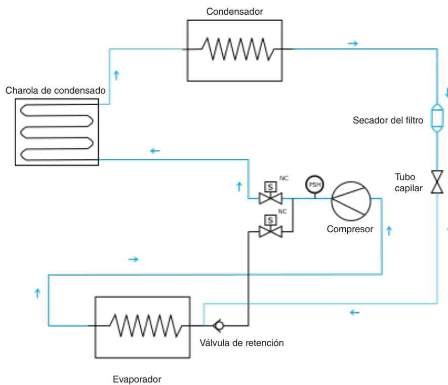
Diagrama del sistema - Modo de refrigeración (FNGSC4A)
