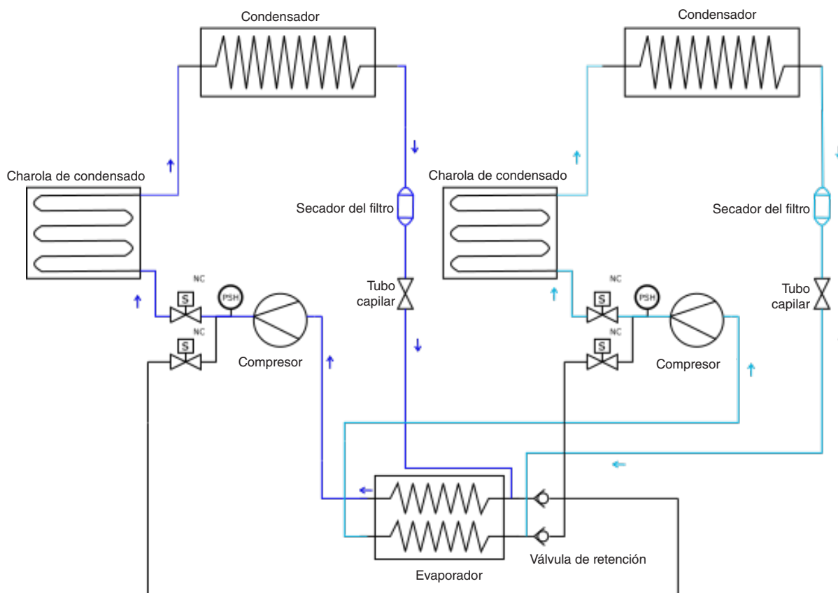
Diagrama del sistema - Modo de refrigeración (FNGSC8A)
