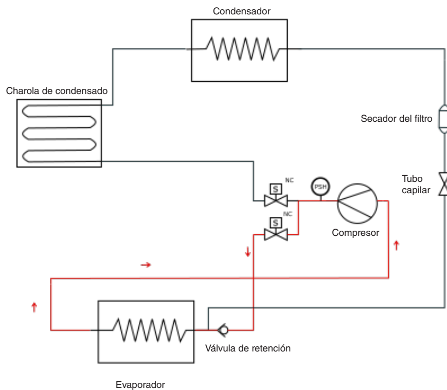
Diagrama del sistema — Modo de deshielo —Derivación de gas caliente (FNGSC4A)
