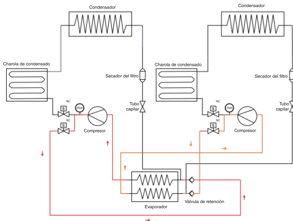
Diagrama del sistema — Modo de deshielo — Derivación de gas caliente (FNGSC8A)
