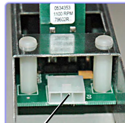
Señal de bajo voltaje (3 entradas) al motor de los ventiladores (para la velocidad en RPM)
