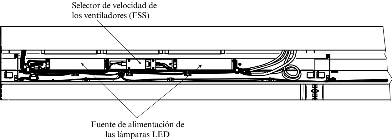
Paso del arnés de cables del selector de velocidad de los ventiladores Exhibidores de un nivel IC2, IC2X IC3 (cuando se requiera)
