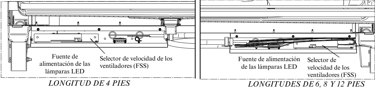
Paso del arnés de cables del selector de velocidad de los ventiladores Exhibidores de un nivel IM1-IP1-IC1 (cuando se requiera)
