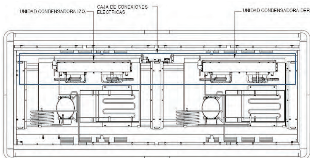
Figura A. Distribución del compartimento de la maquina (se muestra el gabinete de 8 pies)
