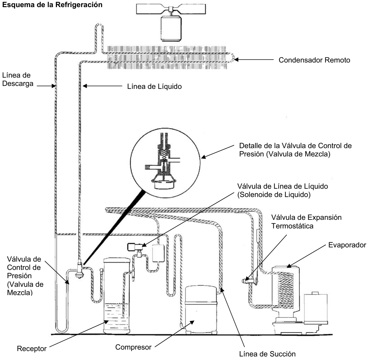
Esquema de la Refrigeración
