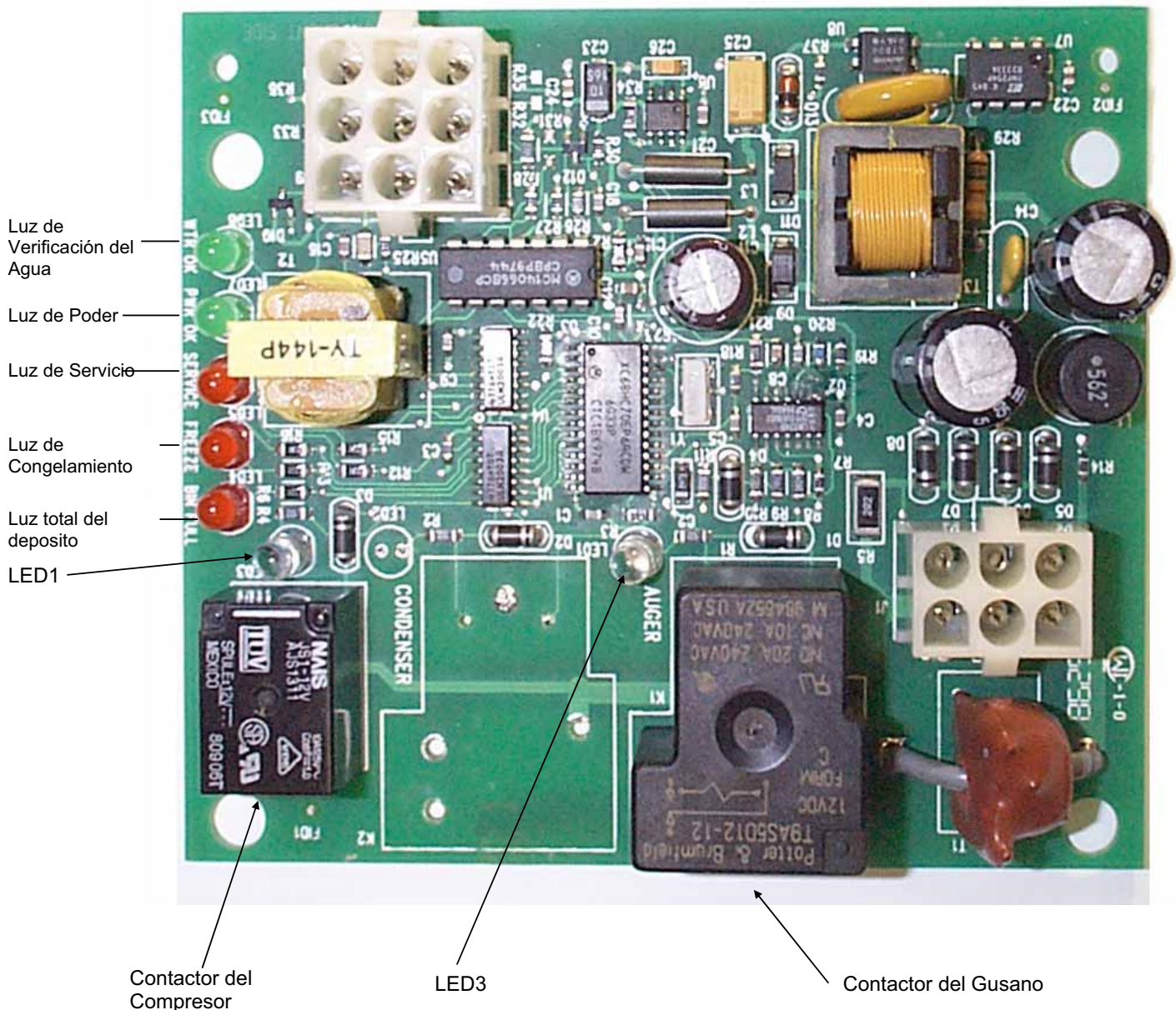
Tarjeta de Control
