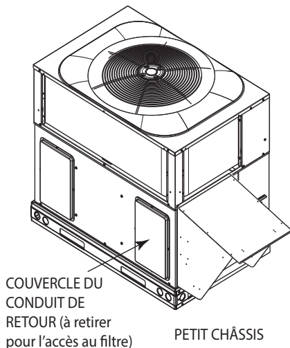
Fig. 8 – Accès au filtre à petit châssis
