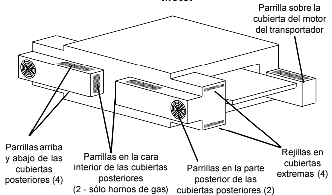
Figura 4-2 - Rejillas posteriores y rejilla del protector del motor
