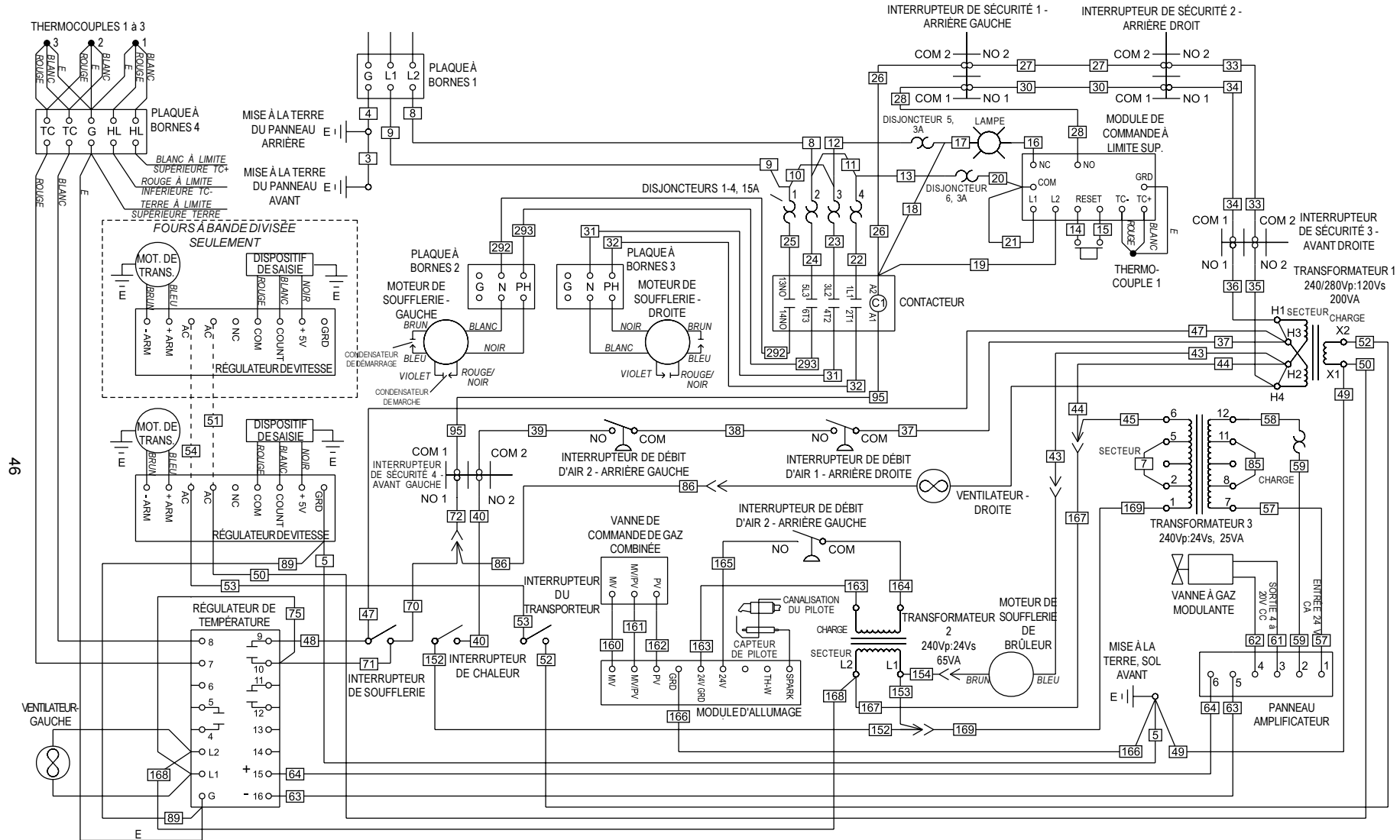
Fig. 5-1 Schéma de câblage, fours à gaz PS555G ou PS570G, 208/240 V, 50/60 Hz, 1 Ph
