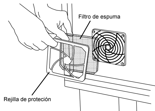
Figura 4-2 - Rejillas posteriores y rejilla del protector del motor
