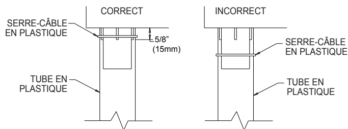
DÉTAIL A
