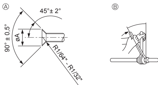
A Dimensiones del corte abocinado B Torsión de apriete de la tuerca abocardinada
