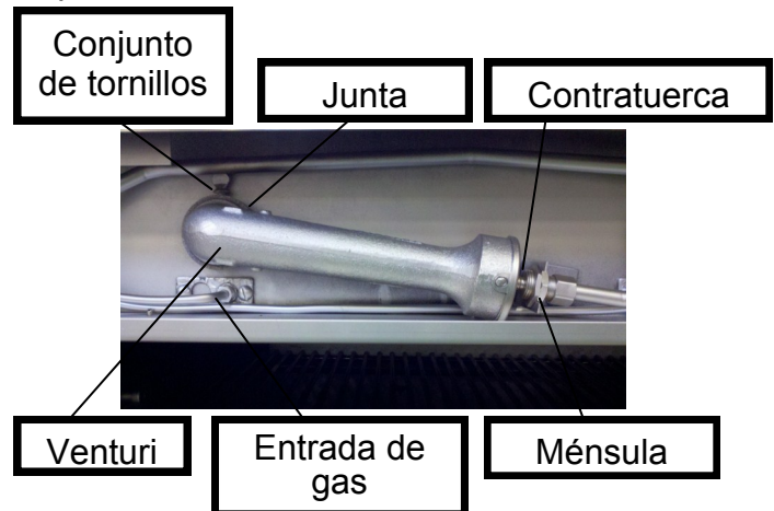
Figura 8. Conjunto de quemador piloto
