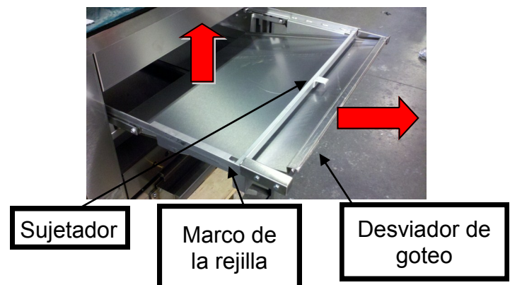
FIGURA 3. DESVIADOR DE GOTEO
