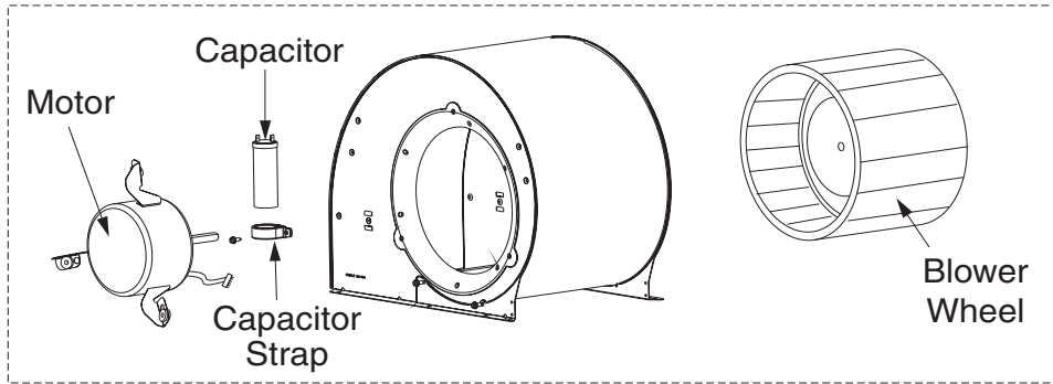
5 Ton Blower
