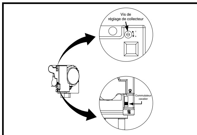
Figure 21. Vanne modulatrice à gaz
