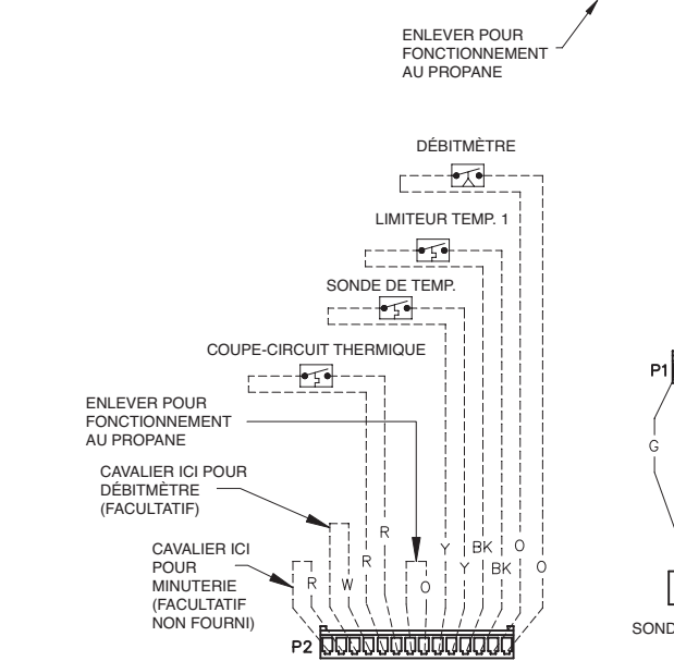
Figure 36. Câblage modèle P-156
