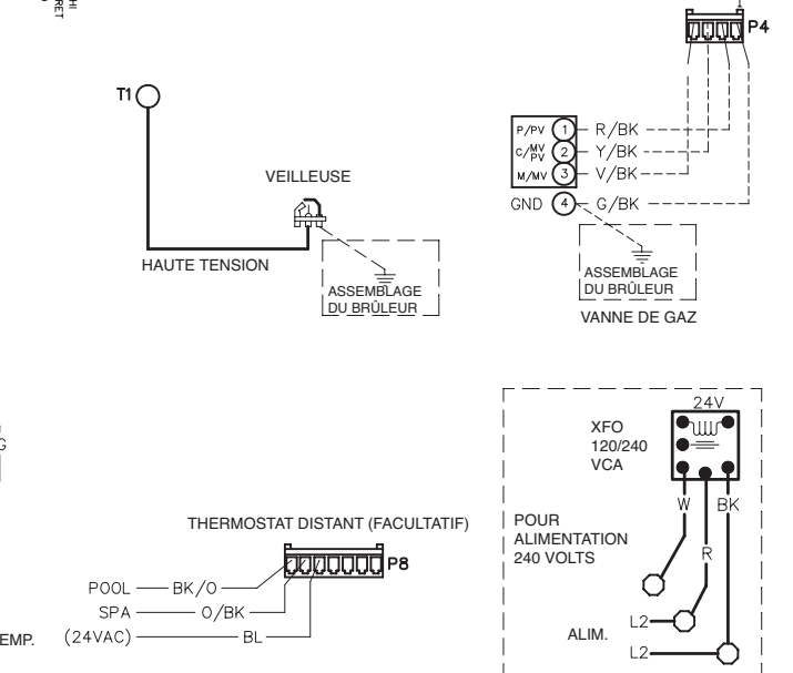
Figure 36. Câblage modèle P-156
