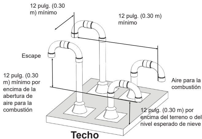
Figura 32: Terminación vertical de tubería doble de calentadores de agua múltiples
