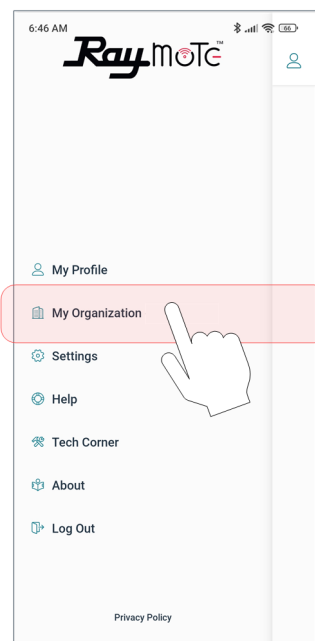
Figure 133. Menu utilisateur
