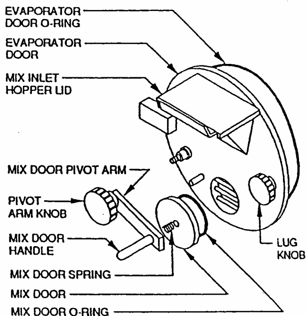
Fig. 2-A Door Assembly (B-10, B-20, B-48)
