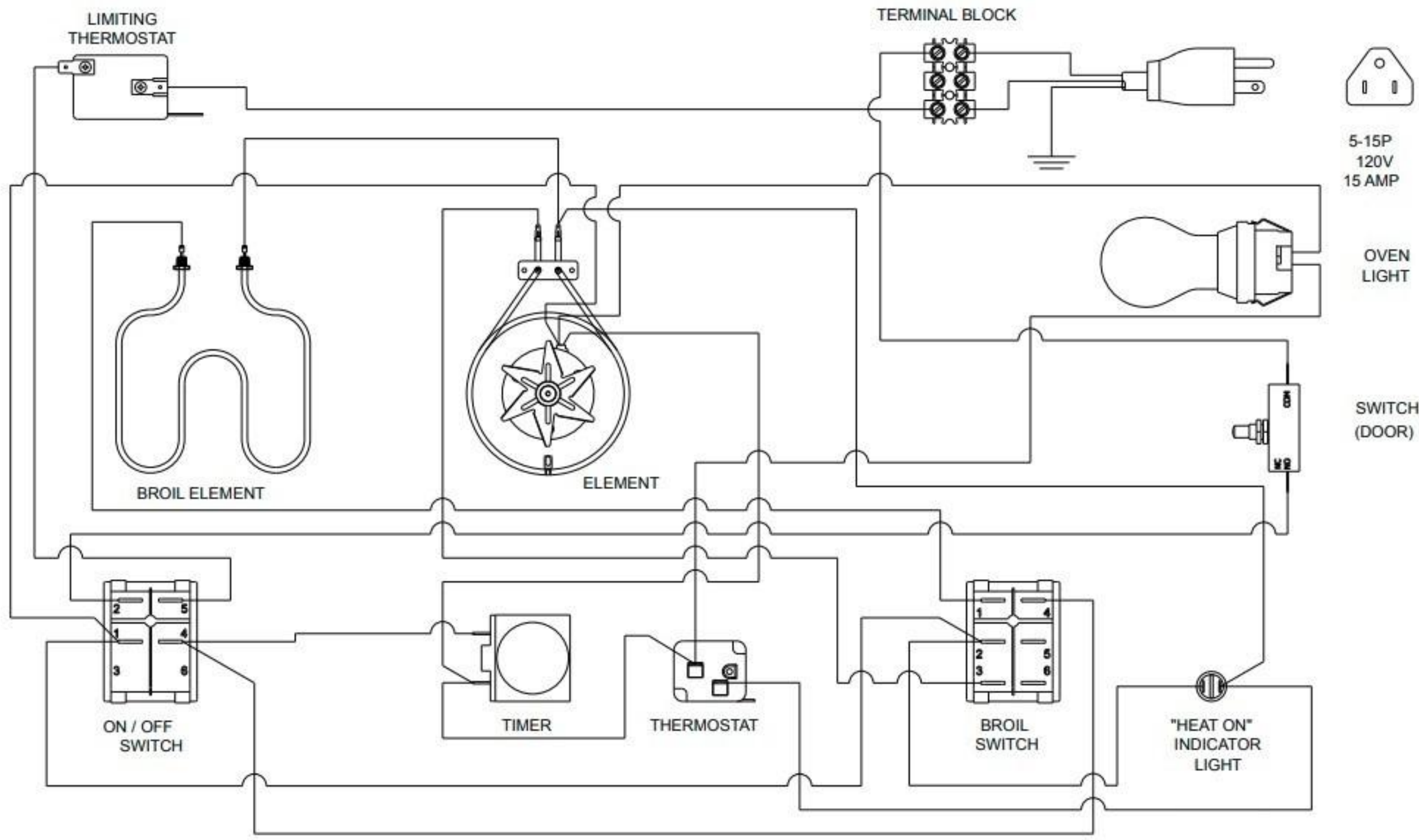
WIRING SCHEMATIC
