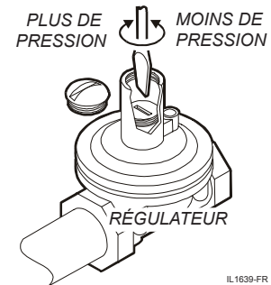
Fig. 3 Réglage de la pression du gaz
