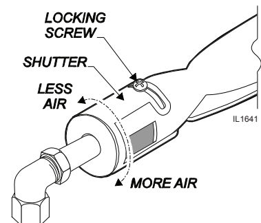
Fig. 5 Réglage de la flamme du brûleur
