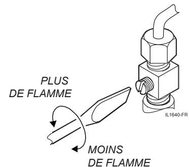
Fig. 4 Réglage de la flamme de la veilleuse
